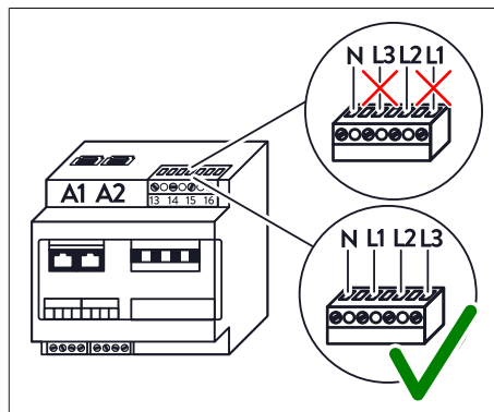
Abb. 9: Anschluss Spannungsmessung
