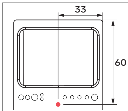
Abb. 3: Position für Leitungsdurchführung (Abbildung nicht maßstabsgetreu - alle Angaben in Zentimetern)
